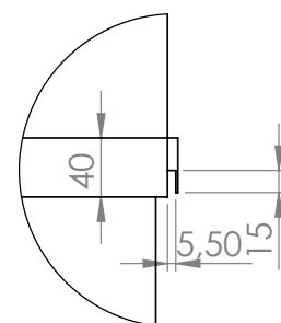
Accroche machine
