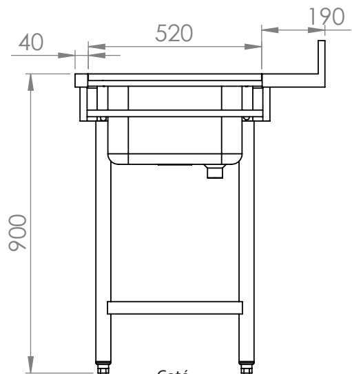
Coté
