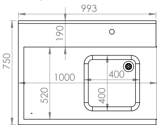
Dessus
